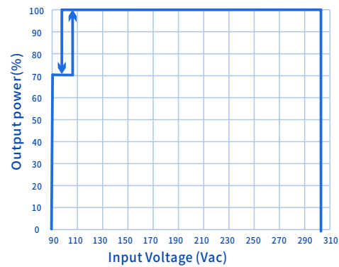
降额曲线（输出功率Vs.输入电压）
